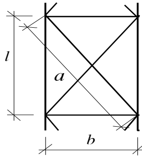
Hình 6 – Sơ đồ thanh giằng chữ thập
