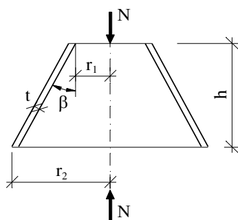
Hình 17 – Sơ đồ vỏ nón tròn xoay chịu lực nén dọc trục
